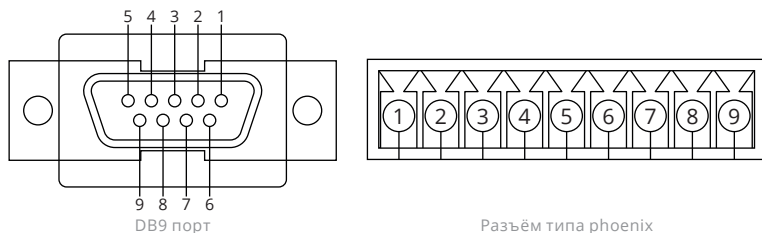
Рис. 5-1: Сухие контакты
