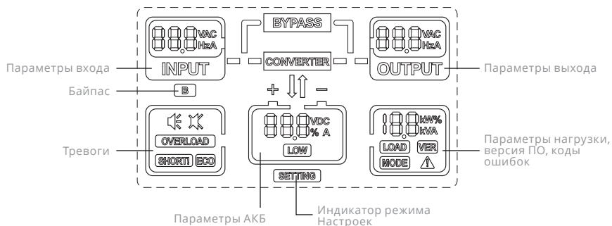
Рис. 3-2: Меню ЖК-дисплея
