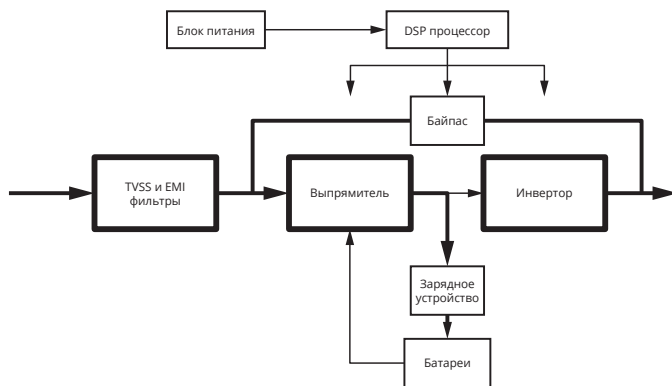
Рис 1-5: Режим байпаса
