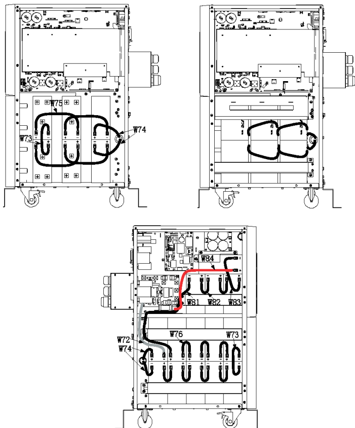
Схема размещения 20-ти АКБ в стандартной модели 6000 ВА.
