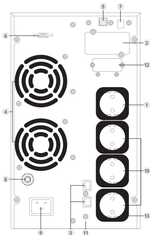
Рис. 3: Вид сзади: ИБП ИМПУЛЬС СПРИНТЕР11-2 (2 кВА) и ИБП ИМПУЛЬС СПРИНТЕР11-3 (3 кВА)
